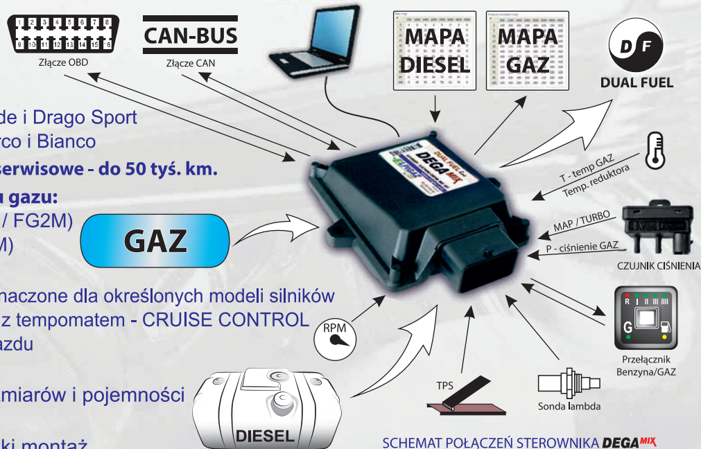
SCHEMAT POŁĄCZEŃ STEROWNIKA DEGA MIX
